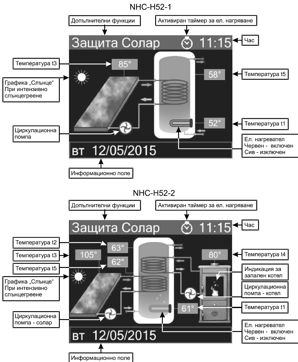
Фиг. 4 - Дисплей на електронни блокове NHC-H52-1 / NHC-H52-2
