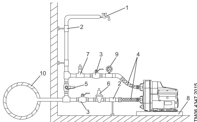
Фиг. 5 Усилване на налягането на водата в главния водопровод
