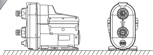
Фиг. 1 Хоризонтален фундамент
